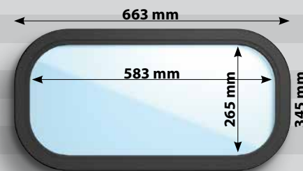
Abgerundete Ecken ( r = 120 \text{ mm} ), hoher Isolierungswert
